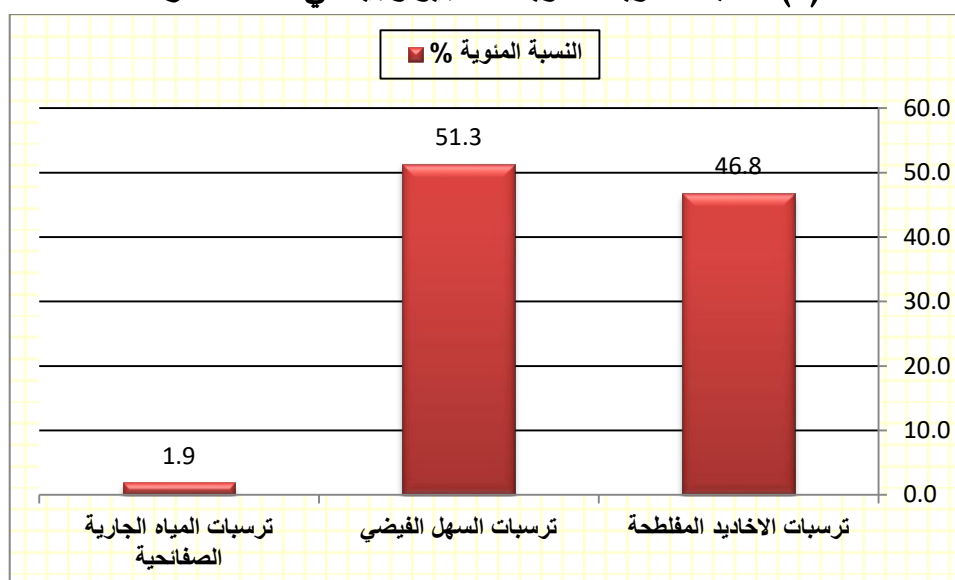
شكل (1) النسبة المئوية للتكوينات الجيولوجية في منطقة الدراسة .
