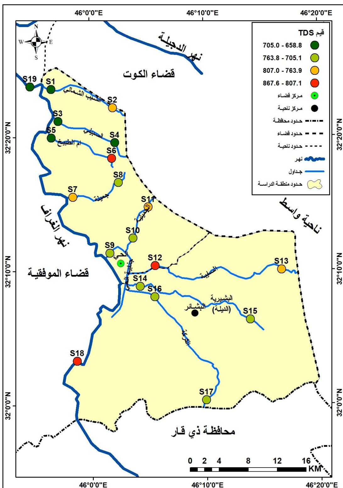
خريطة (13) قيم الأملاح الذائبة TDS في منطقة الدراسة .
