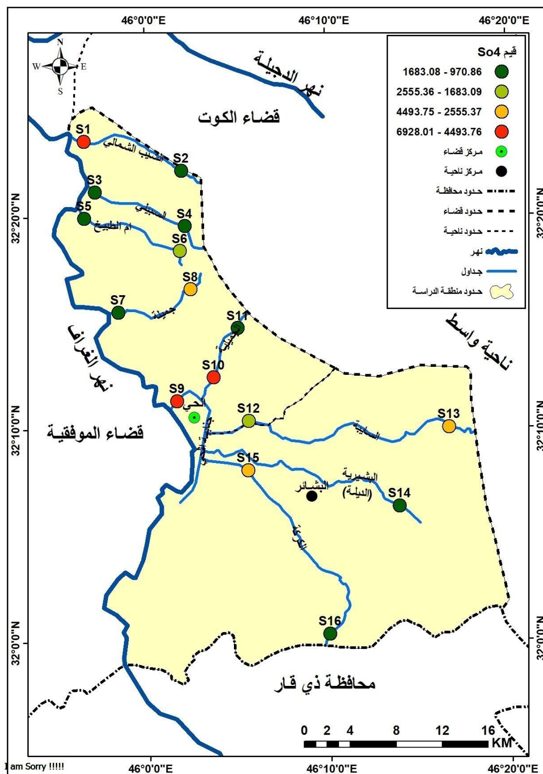
خريطة (39) قيم أيون الكبريتات SO_4 للتراب في منطقة الدراسة .
