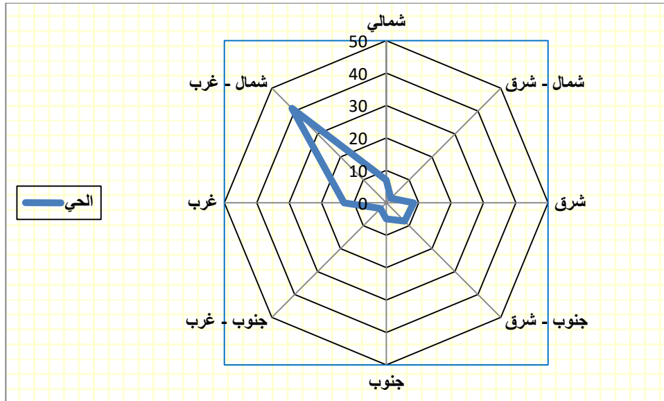
الشكل (12) ورده الرياح لمحطة الحي المناخية .
