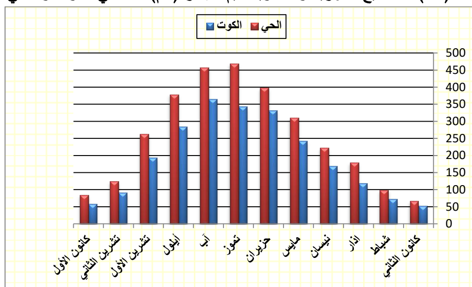
الشكل (15) المجاميع الشهرية و السنوية لقيم التبخر (ملم) لمحطتي الكوت و الحي .
