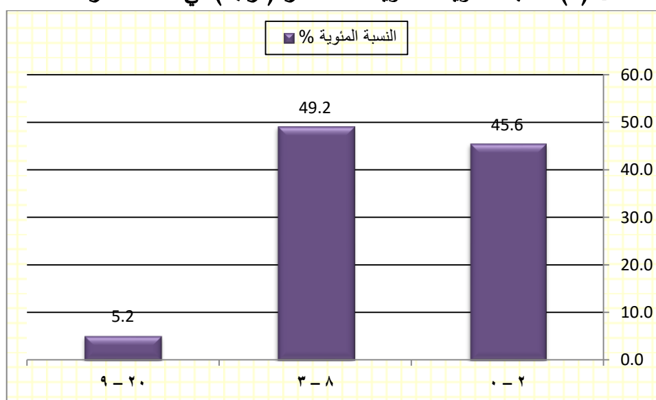
شكل (3) النسبة المئوية لمستويات الانحدار (درجة) في منطقة الدراسة .
