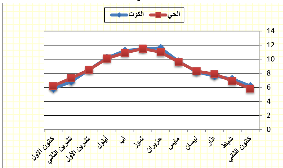
الشكل (5) المعدلات الشهرية لساعات السطوع الشمسي الفعلي ساعة / يوم لمحطتي الكوت و الحي.
