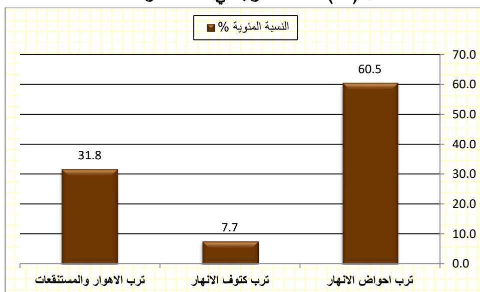
شكل (16) أصناف الترب في منطقة الدراسة .
