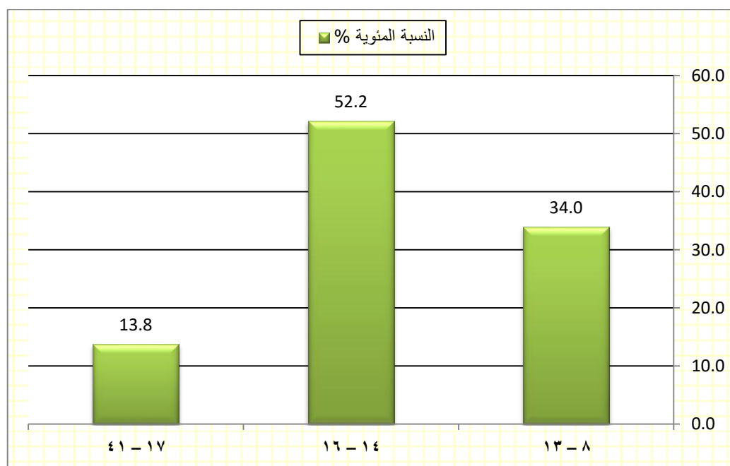
شكل (2) النسبة المئوية لفئات الارتفاع (متر) في منطقة الدراسة .
