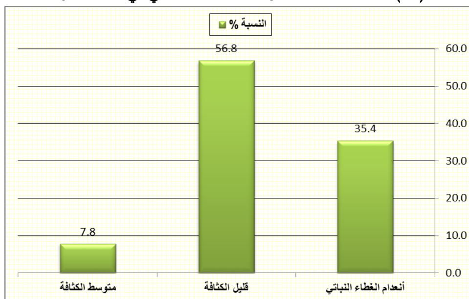
شكل (17) النسب المئوية لمؤشر كثافة الغطاء النباتي في منطقة الدراسة .
