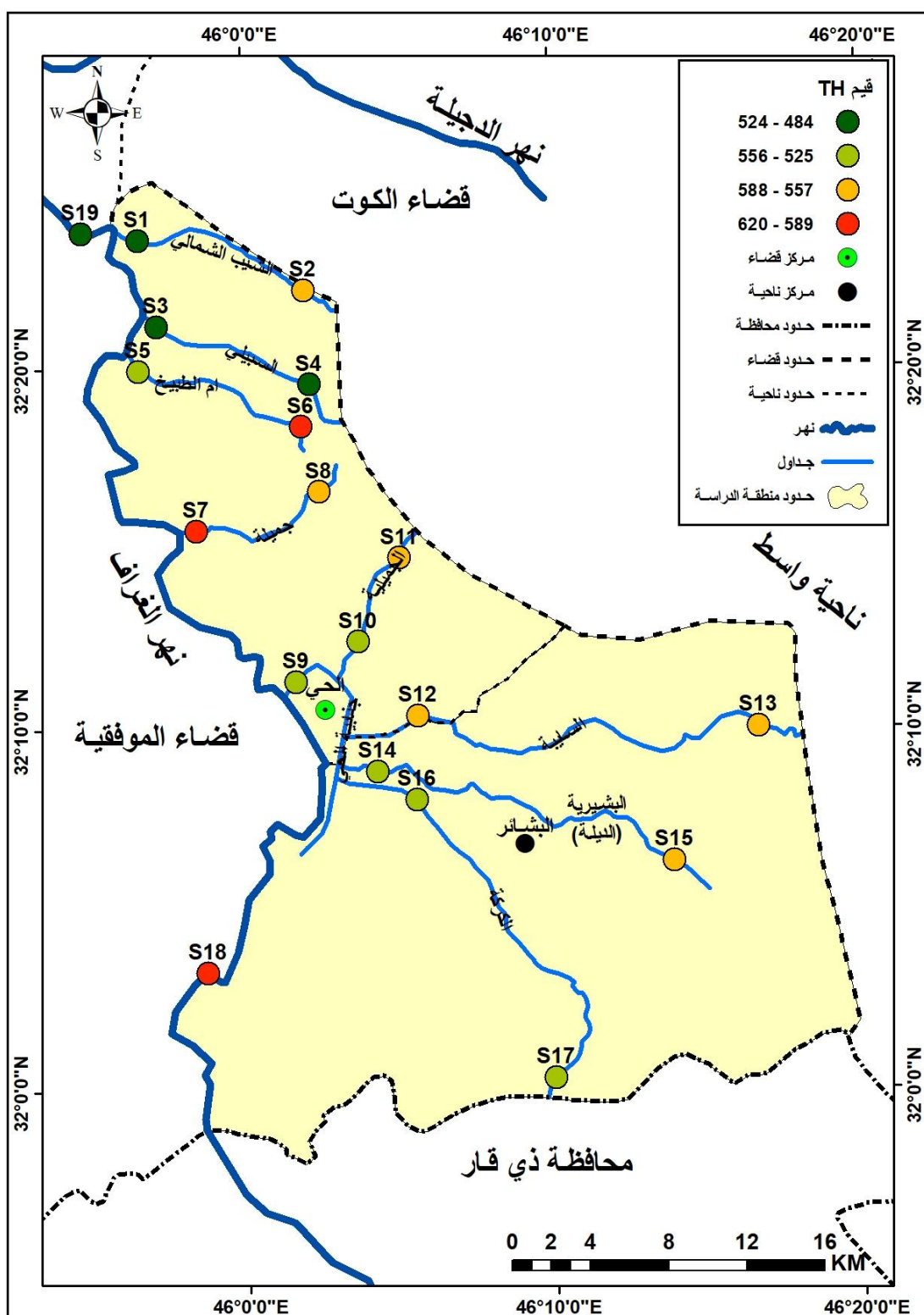
خريطة (11) قيم العسرة الكلية TH في منطقة الدراسة .
