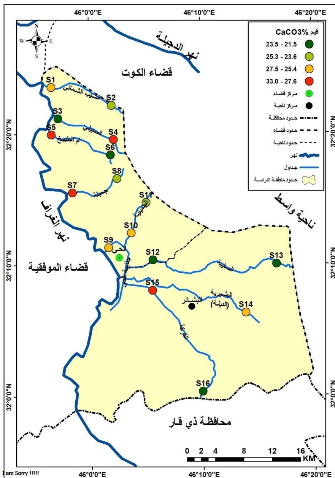
خريطة (42) قيم أيون كبريتات الكالسيوم للترب في منطقة الدراسة .
