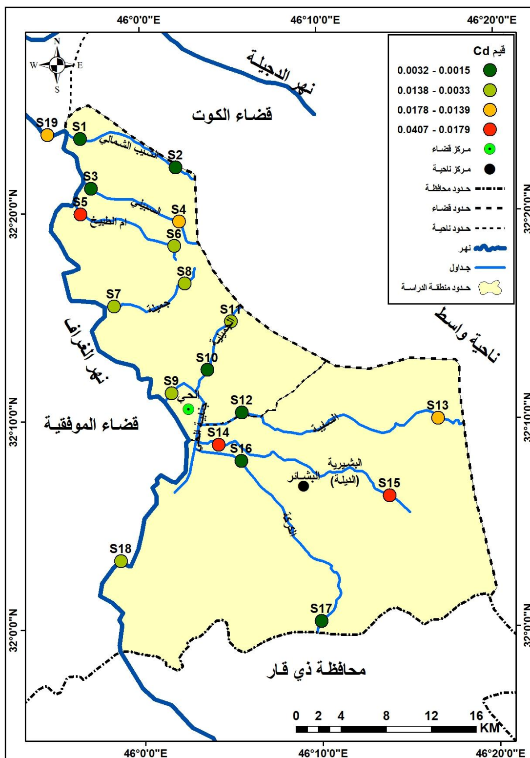
خريطة (26) قيم عنصر الكاديوم Cd للمياه في منطقة الدراسة .
