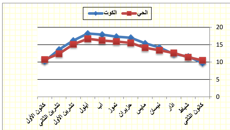
الشكل (8) المعدلات الشهرية للمدى الحراري (م) لمحطتي الكوت و الحي للمدة من (2014 – 2024) .
