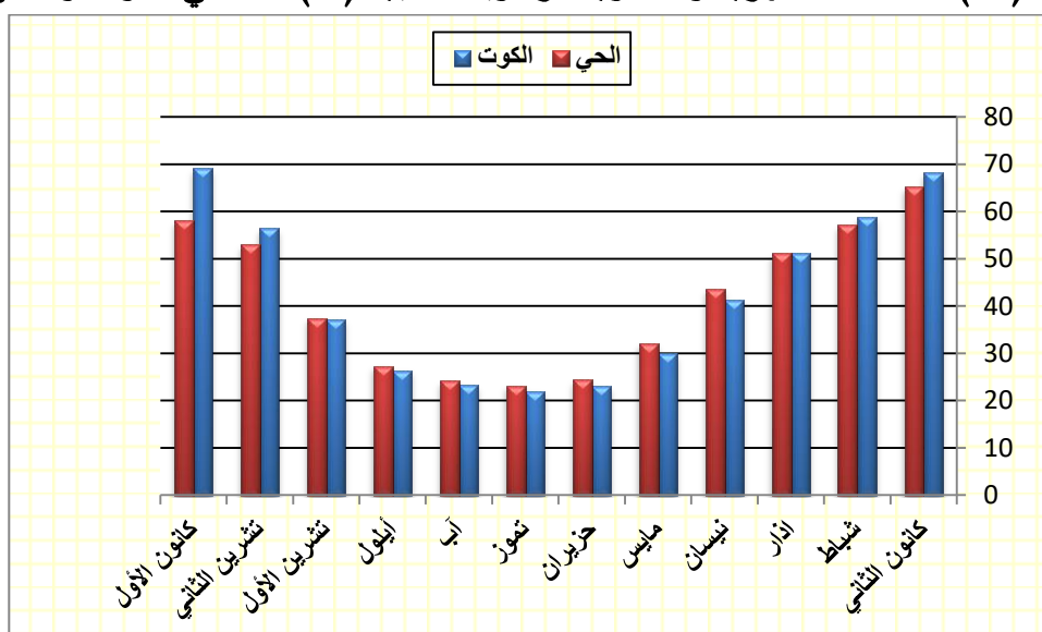
الشكل (14) المعدلات الشهرية و السنوية للرطوبة النسبية (%) لمحطتي الكوت و الحي .
