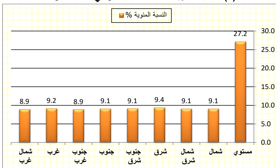
شكل (4) النسب المئوية لاتجاهات الانحدار في منطقة الدراسة .
