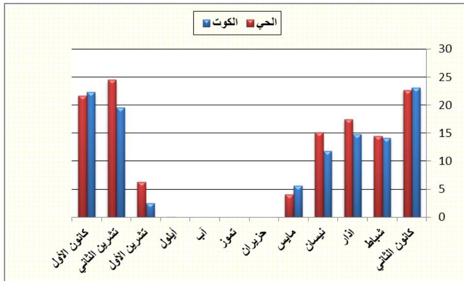
الشكل (13) المعدلات الشهرية و السنوية للأمطار (ملم) في محطات منطقة الدراسة للمدة من (2014 - 2024) .
