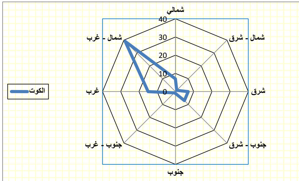
الشكل (11) ورده الرياح لمحطة الكوت المناخية .
